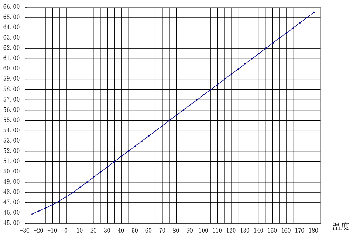
温度—阻值曲线图
