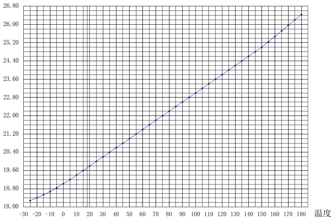
温度—电阻对应表
